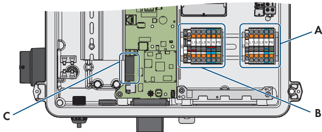
Figura 10: Punti di collegamento all'interno del prodotto
