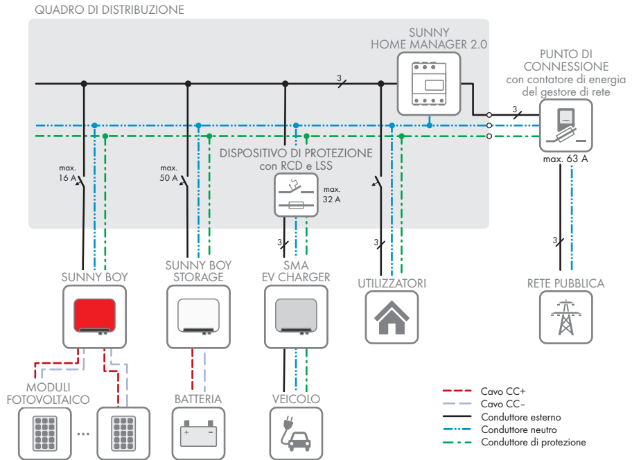
Figura 4: Panoramica dei collegamenti (esempio con EVC22-3AC-10)
