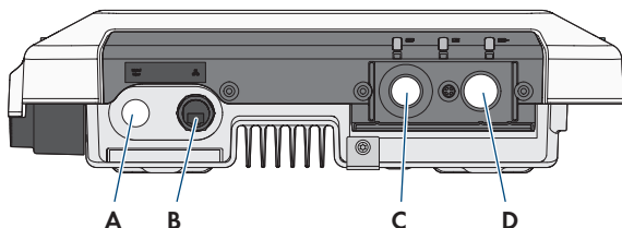
Figura 9: Vista dal basso del prodotto con coperchio del campo di collegamento installato
