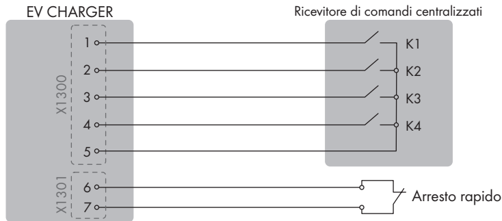
Figura 12: Collegamento di un ricevitore di comandi centralizzati
