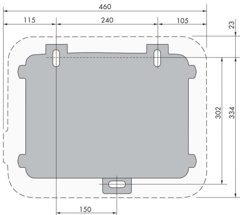
Figura 7: Posizione dei punti di fissaggio (Misure in mm/in)
