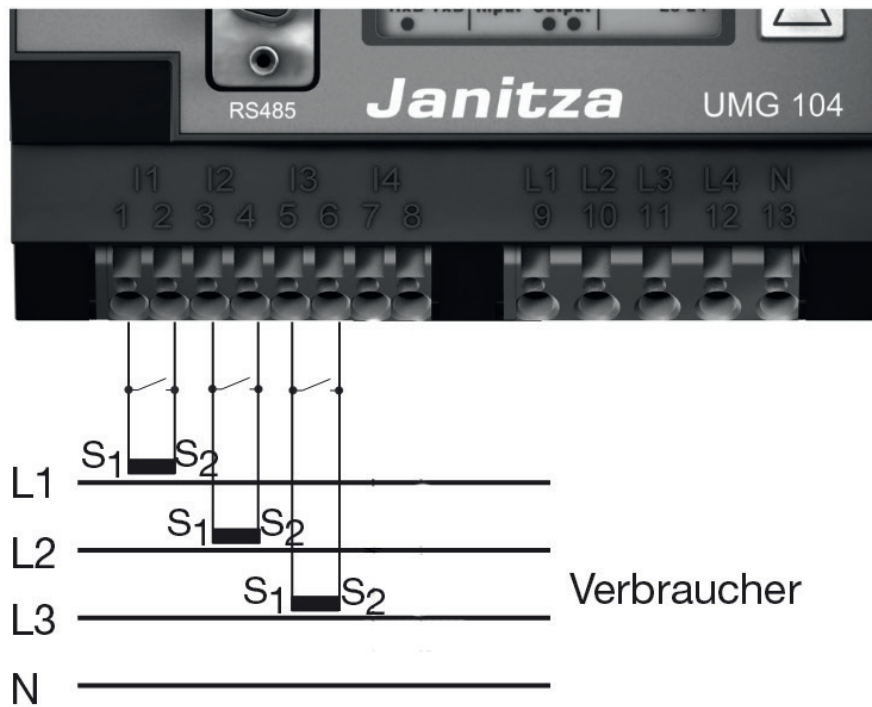
Abb.: Anschlusschema Strommessung Utility Meter mit Messwandlern
