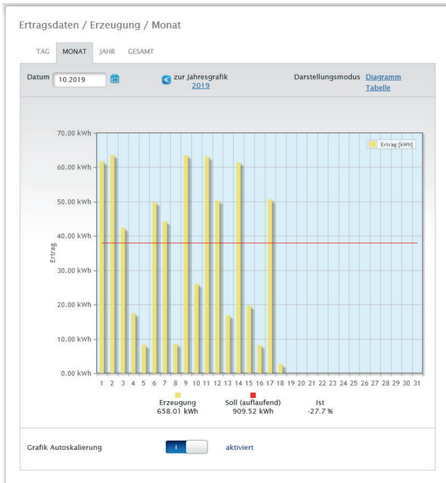
Abb.: Diagramm Monats-Ansicht
