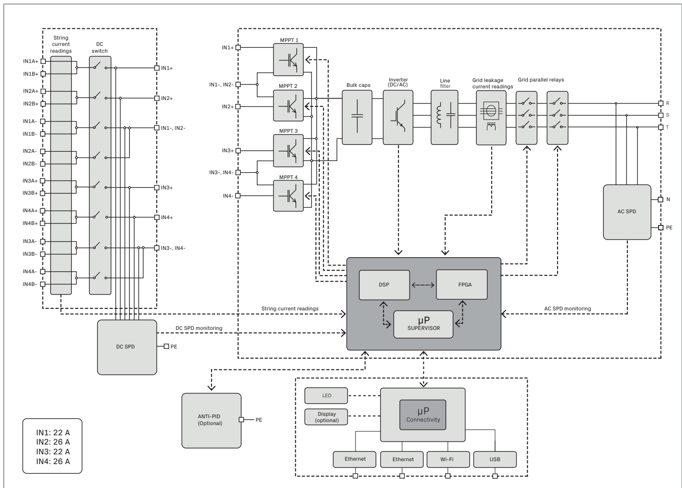
Diagramma a blocchi PVS-20-30-33-TL
