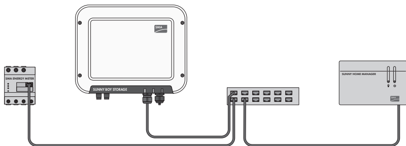
Figura 11: Collegamento di rete in Flexible Storage System con Sunny Home Manager (esempio)
