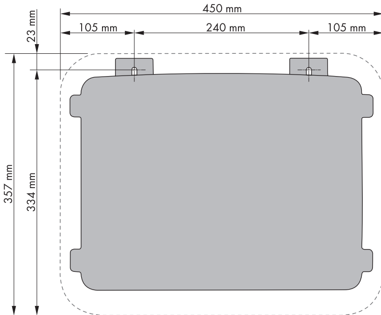
Figura 6: Posizione dei punti di fissaggio
