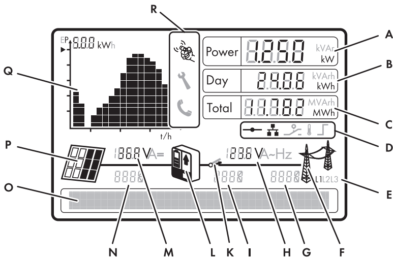
Figura 13: Struttura del display (esempio)
