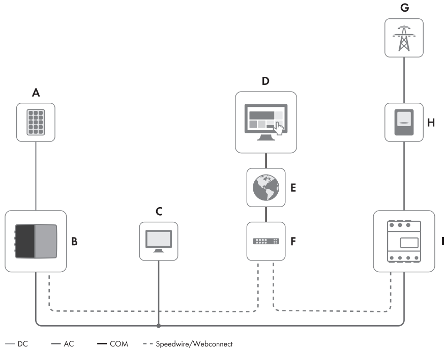
Figura 4: Panoramica di un sistema con Sunny Boy Smart Energy, Battery Pack e SMA Energy Meter (esempio)
