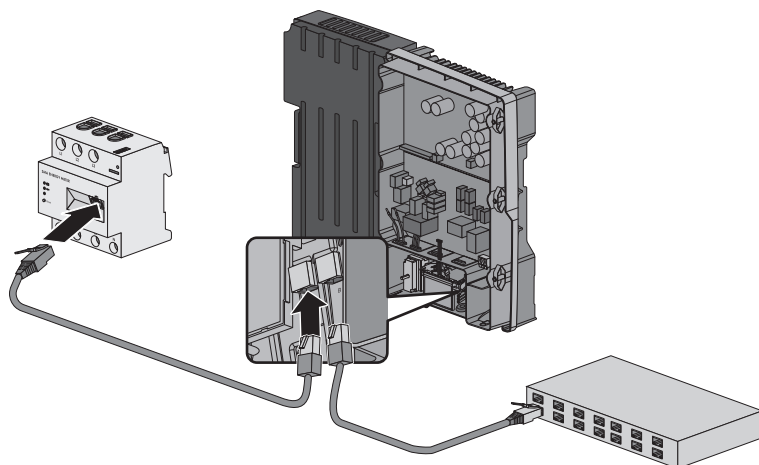
Figura 11: Variante di collegamento con Sunny Boy Smart Energy e SMA Energy Meter (esempio)
