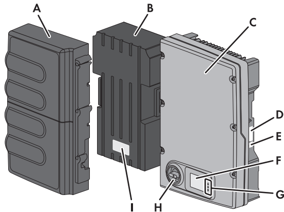
Figura 2: Struttura di Sunny Boy con Battery Pack
