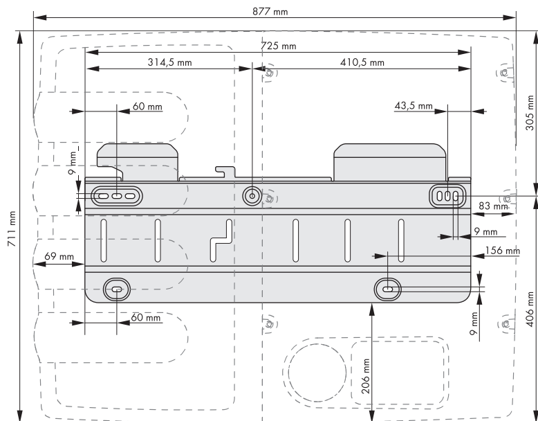
Figura 5: Dimensioni del supporto da parete
