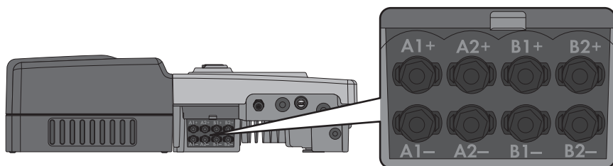
Figura 12: Panoramica degli ingressi CC sull'inverter
