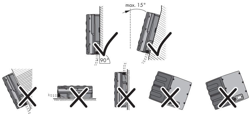
Figura 7: Posizioni di montaggio consentite e non consentite
