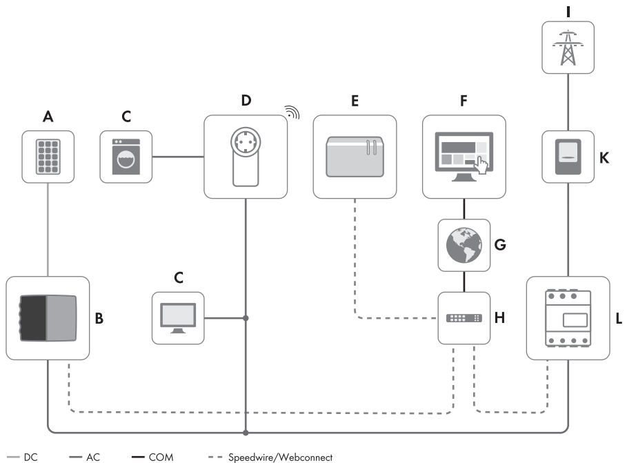
Figura 3: Panoramica di un sistema di accumulo integrato (esempio)
