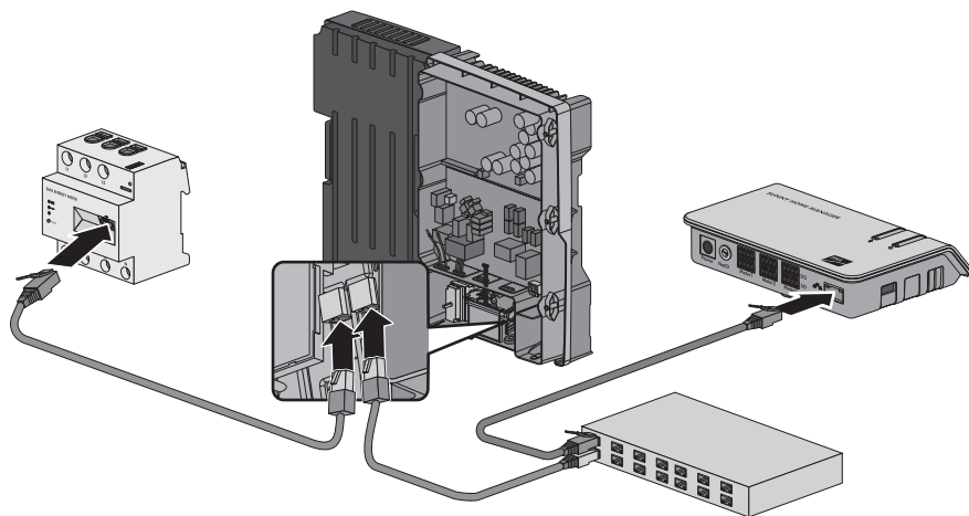
Figura 10: Variante di collegamento con sistema di accumulo integrato (esempio)
