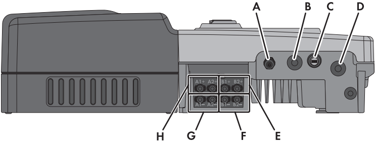
Figura 8: Punti di collegamento e aperture sul fondo dell'inverter
