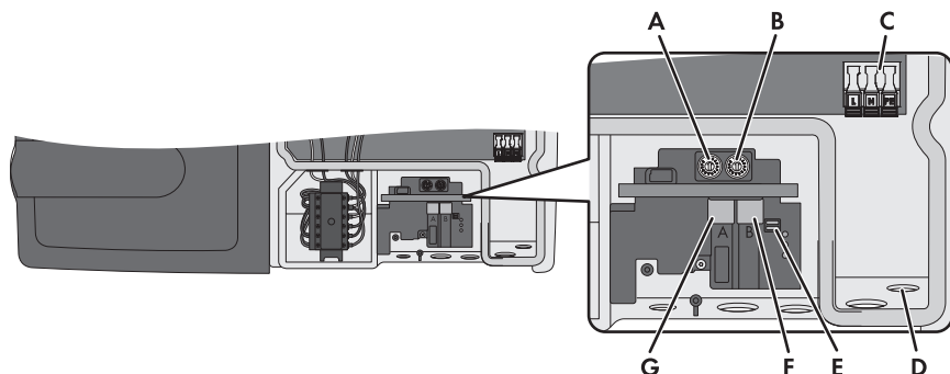
Figura 9: Punti di collegamento all'interno dell'inverter
