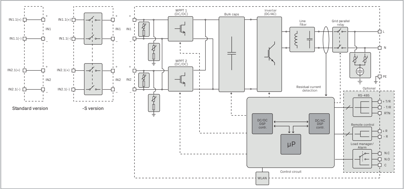
Diagramma a blocchi UNO-DM-3.3/4.0/4.6/5.0-TL-PLUS-Q
